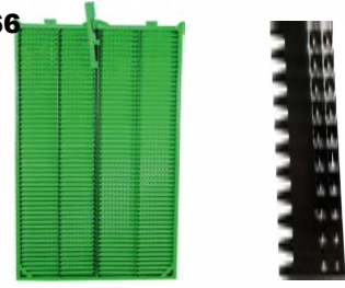
UCZ-12765 (AZ46424) LOWER SIEVE 1230X1520 (1174)
