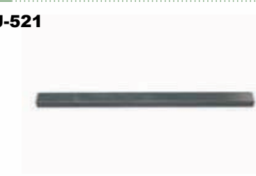
UCZ-1930 KEY - (12x8x200mm) (955)
